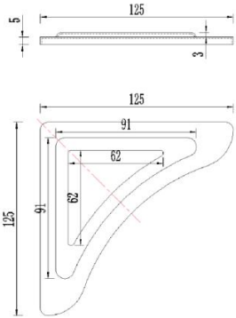
样品 6、床横梁下方三角形加固件小样 (未喷漆 1 个)：横梁下方设计三角形加固件，规格 125mm×125mm，外侧面为弧形设计，内设计两个外形接近三角形的加强筋设计，两边长各不小于 90mm、60mm。如下图所示。
