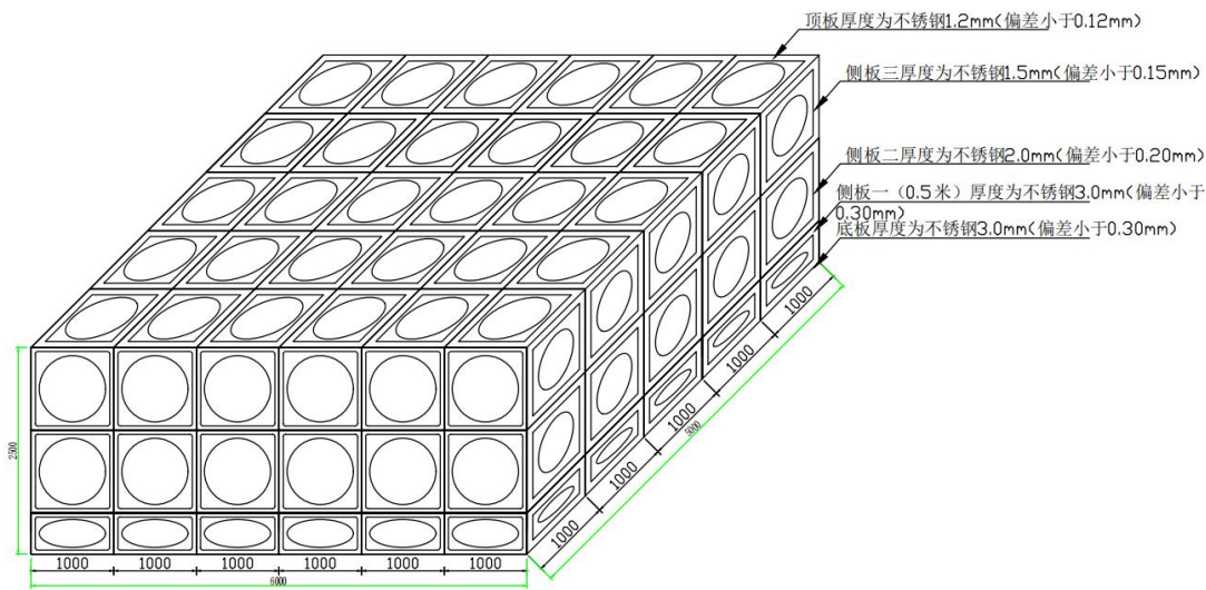
HYBX不锈钢生活水箱6.0m×5.0m×2.5m
