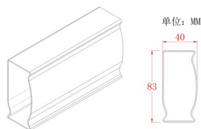
(床厅截面尺寸示意图)
