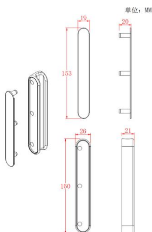
（抽屉拉手示意图）
