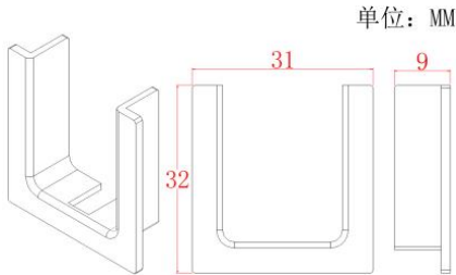
（床厅消音垫尺寸示意图）
