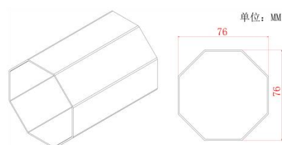
(立柱截面尺寸示意图)
