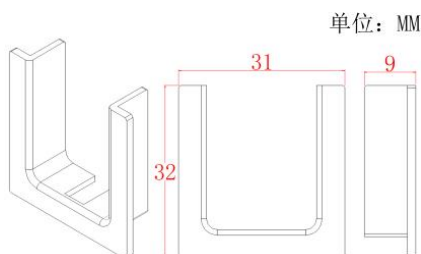
(床厅消音垫尺寸示意图)
