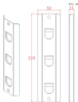
(卡式连接件尺寸示意图)
