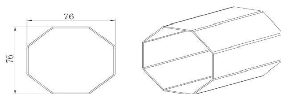
(立柱截面尺寸示意图)
